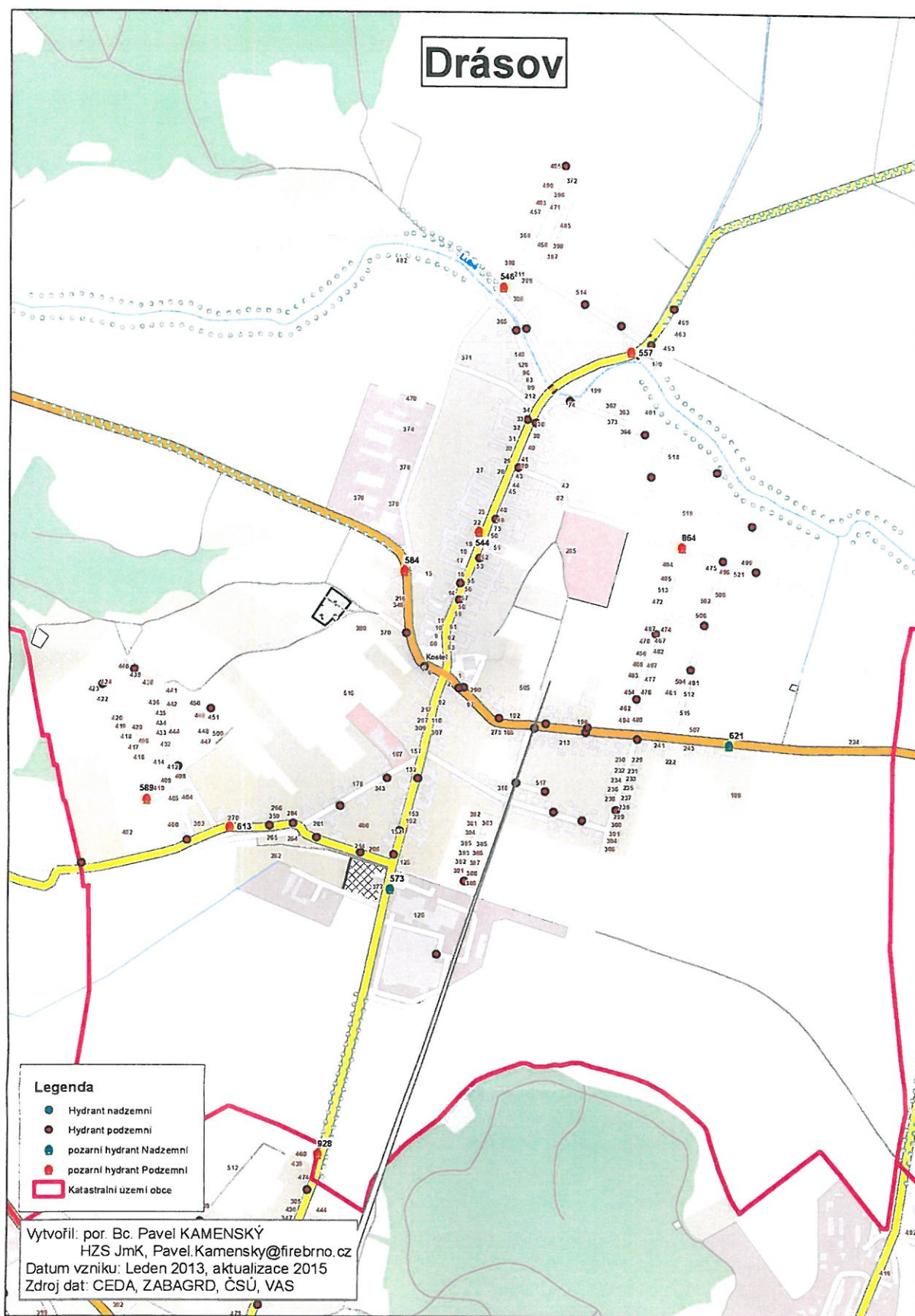
Obrázek č.1 – Hydrantová síť k.ú. Drásov
